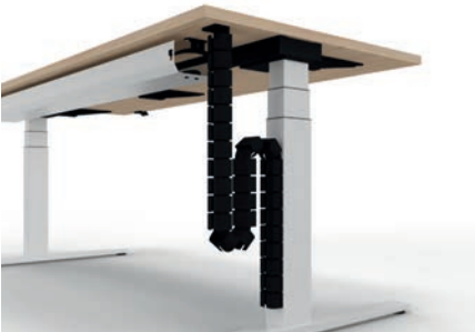
Kabelkette magnetisch an der Säule montiert Cable chain magnetically attached to the column
